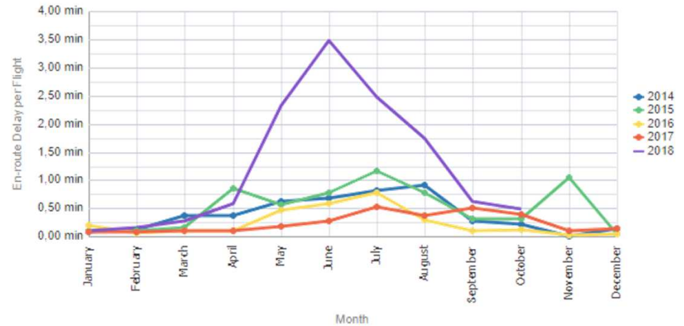
REIMS U/ACC ER Delay per Flight Evolution per Month
